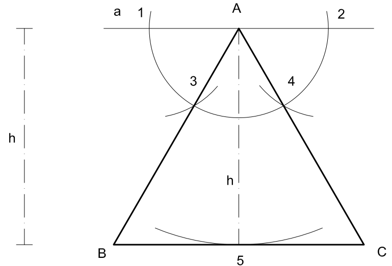
Data l'altezza h , costruire il triangolo equilatero
