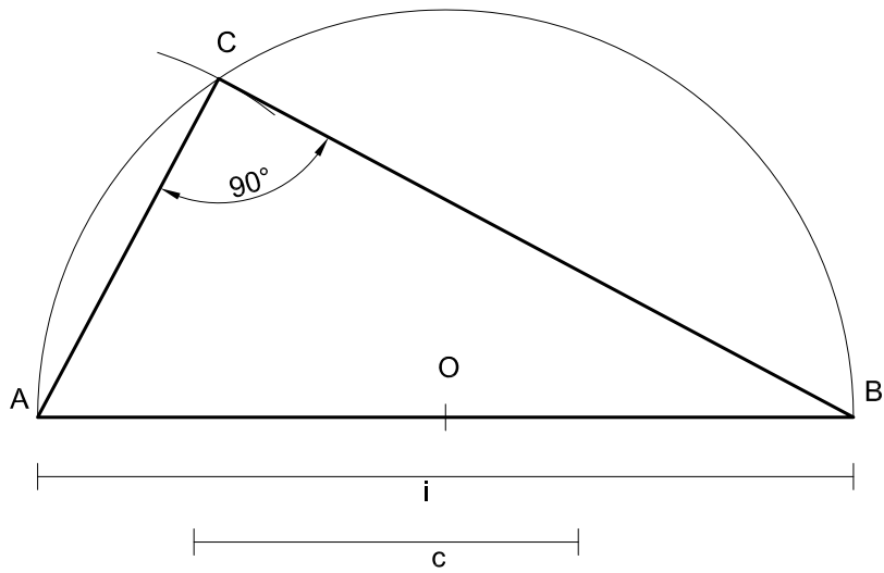
Dati l'ipotenusa a e il cateto c , costruire il triangolo rettangolo
